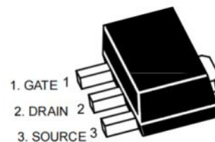
SOT-89-3L
